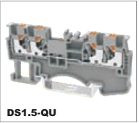
DS1.5-QU 500V/17.5A 0.14-1.5mm 2 UL 300V/15A 26-14AWG T/W/End plate 3.5/63.2/1.5mm
