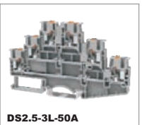
DS2.5-3L-50A 500V/20A 0.2-4mm 2 UL 300V/20A 26-12AWG T/W/End plate 5.2/102/2.2mm
