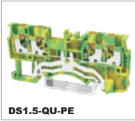
DS1.5-QU-PE — 0.14-1.5mm 2 — 26-14AWG T/W/End plate 3.5/63.2/1.5mm
