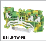
DS1.5-TW-PE — 0.14-1.5mm 2 — 26-14AWG T/W/End plate 3.5/63.2/1.5mm
