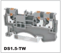
DS1.5-TW 500V/17.5A 0.14-1.5mm 2 300V/15A 26-14AWG T/W/End plate 3.5/54/1.5mm
